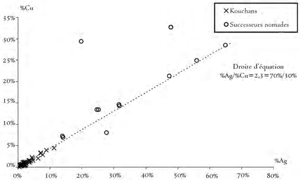
Figure 1: Graphique des teneurs en cuivre en fonction des teneurs en argent, pour toutes les monnaies des Kouchans et de leurs successeurs nomades
